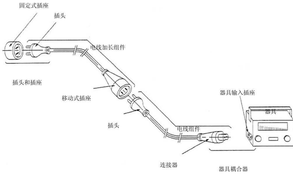
图 1a—各种电器附件及其使用的示意图
