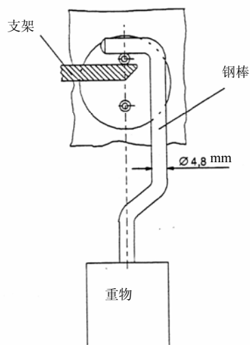
图 14—试验非实心插销的器具
