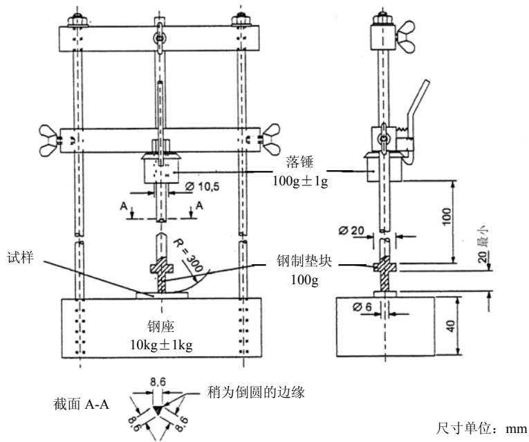
图 42—带有绝缘套的插销的冲击试验装置
