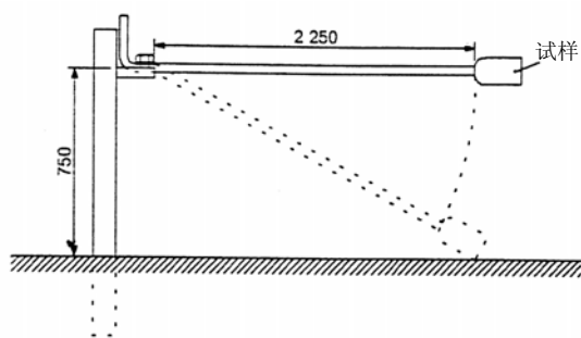
图 29—多位移动式插座机械强度试验装置
