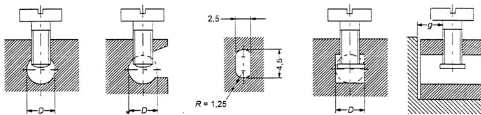
无压力板的端子
