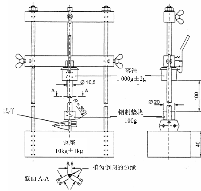
图 27—24.4 的低温冲击试验装置
