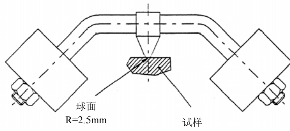
图 37—球压试验装置
