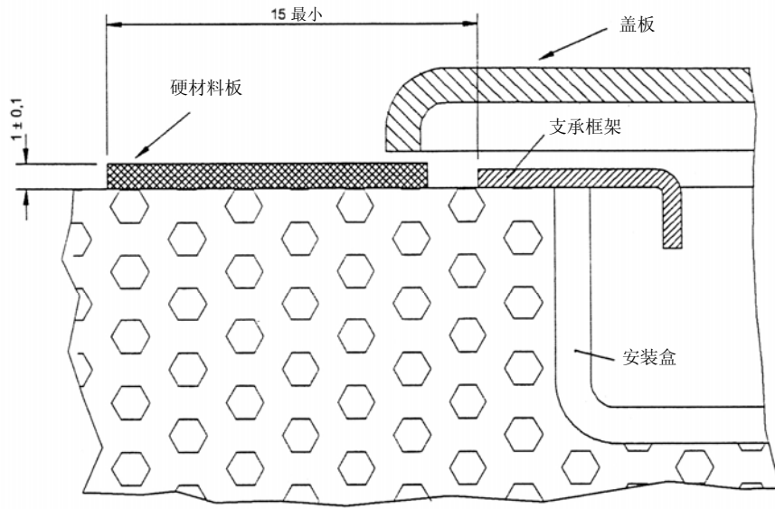
图 31—盖或盖板的试验装置
