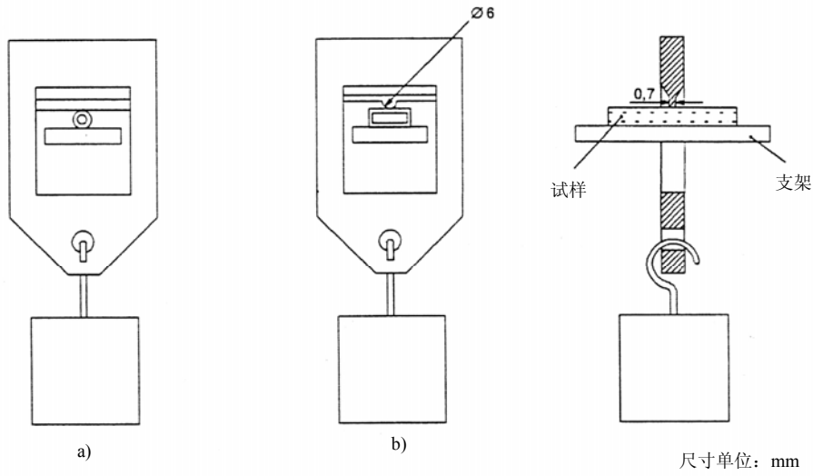
图 41—高温下压力试验装置
