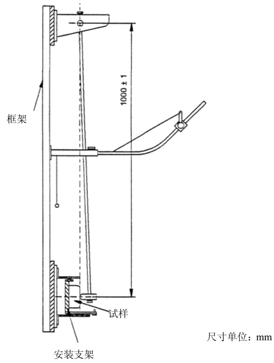
图 22—冲击试验装置
