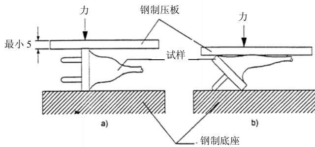
图 8—24.5 的压缩试验装置
